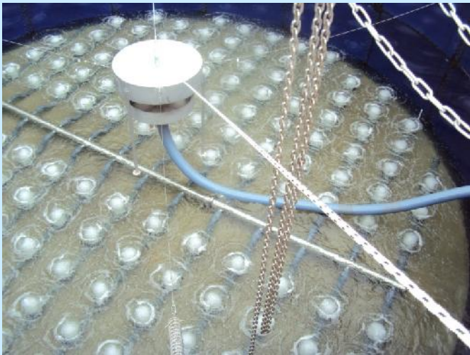
Σύστημα αερισμού και decanter
